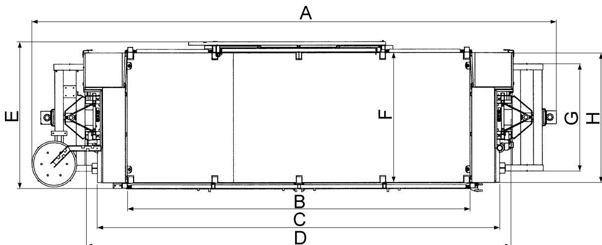
Abb.1-02 Abmessungen oben
