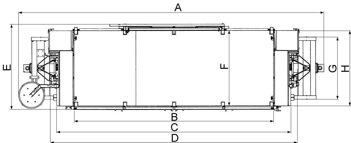
Abb.1-02 Abmessungen oben
